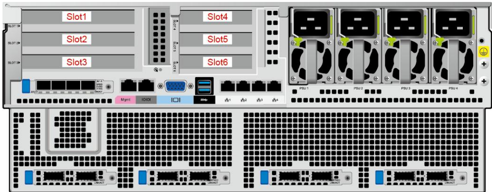
图 4-10 PCIe 插槽位置
