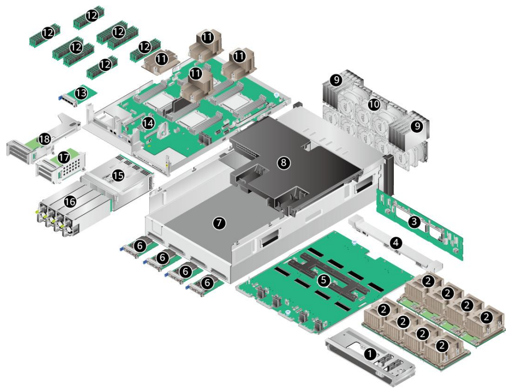
图 3-1 部件示意图
